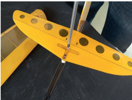
Anschrauben des Höhenleitwerks
